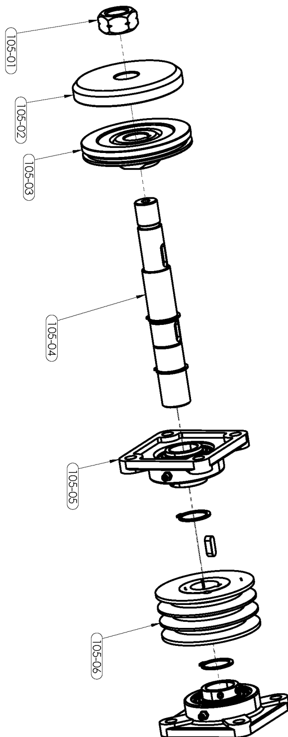
Figura 45 - Unitățile axului acționat
