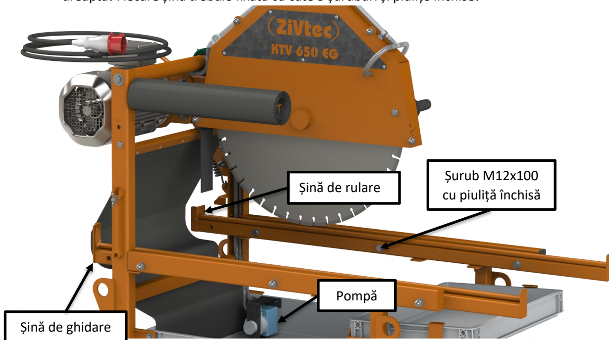
Figura 17 - Montarea/Fixarea șinelor și a pompei
