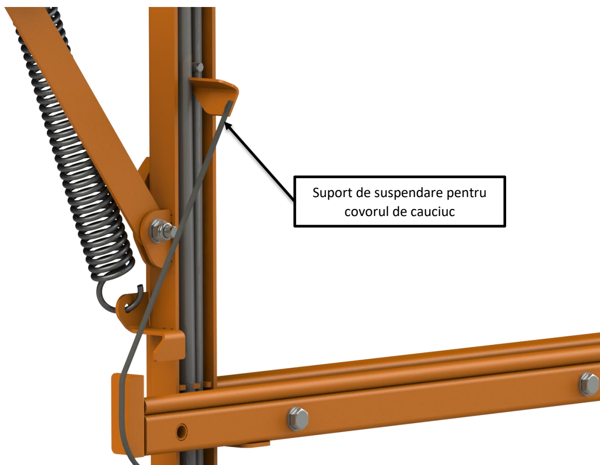
Figura 25 - Fixarea suportului de suspendare pentru covorul de cauciuc 2.
