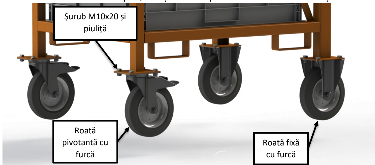
Figura 8 - Montarea roților
