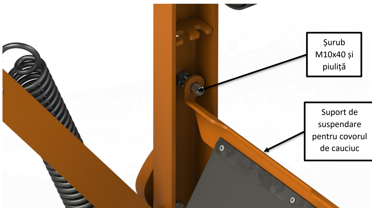
Figura 26 - Fixarea suportului de suspendare pentru covorul de cauciuc 3.
